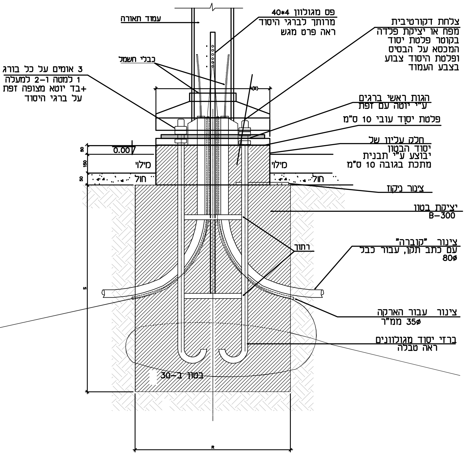
פרט יסוד לעמוד תאורה העומד בגינזון גובה יסוד כגובה קרקע סופיים באותו מקום
