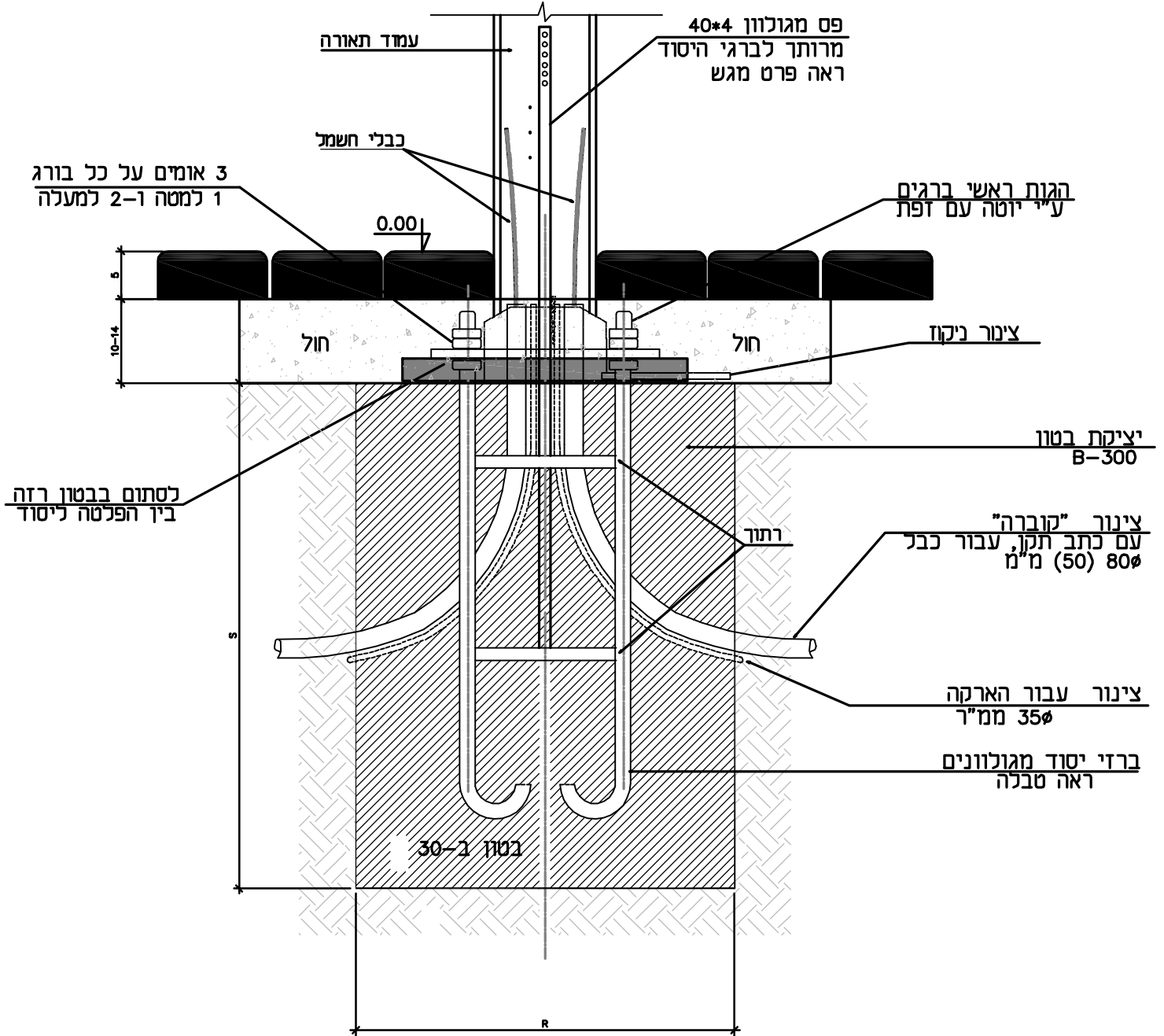
פרט יסוד לעמוד תאורה העומד בריצוף
